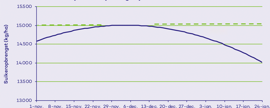
Verloop suikeropbrengst per hectare (2015-2019)
