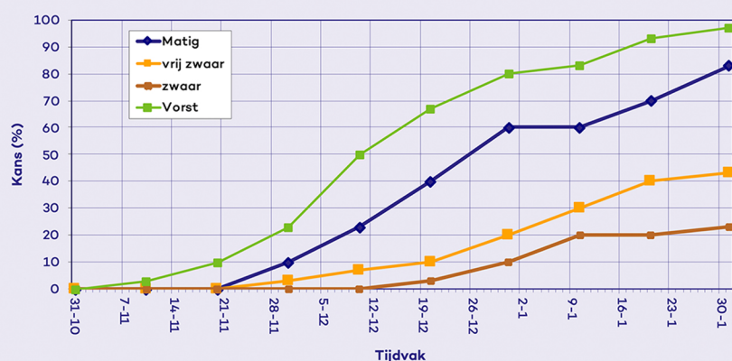
Vorstkansen Nederland tijdens campagne (1991-2020)
